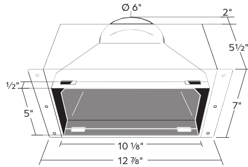
BOÎTE DE GRILLE PW1200200008 Air CHAUD
