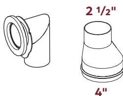
Connecteur pour prise d'air coude 90° Version 16-cube 12002135
