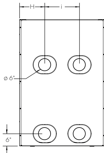
VUE ARRIÈRE
