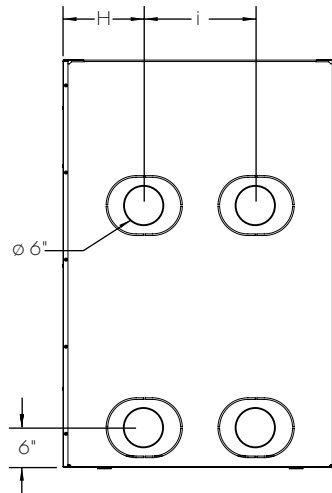
VUE ARRIÈRE
