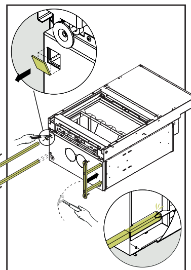
3. Si l'option a été choisie, installer le support ajustable.
