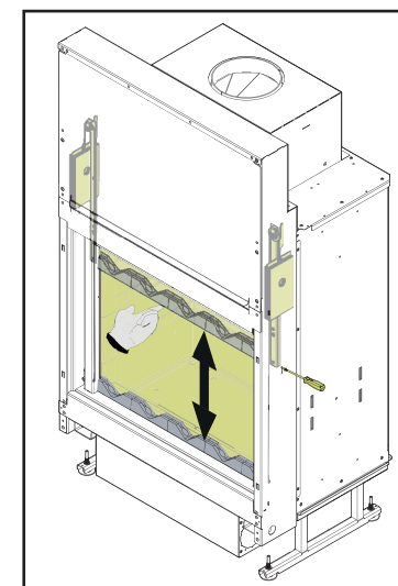
5. Déverrouiller la porte et valider son fonctionnement.
