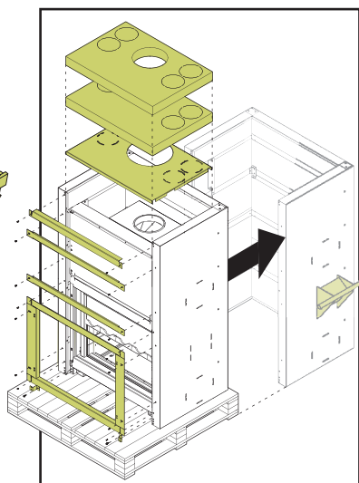
2. Démontez le caisson d'isolation du foyer.
